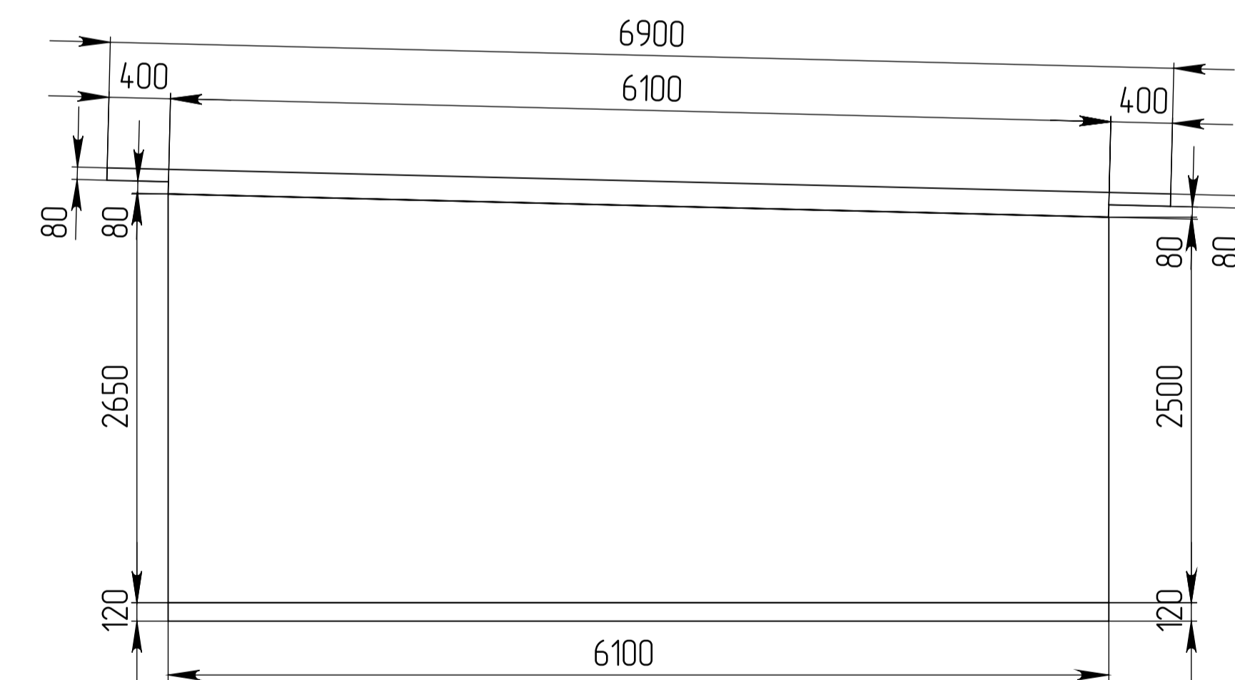
Вид В
